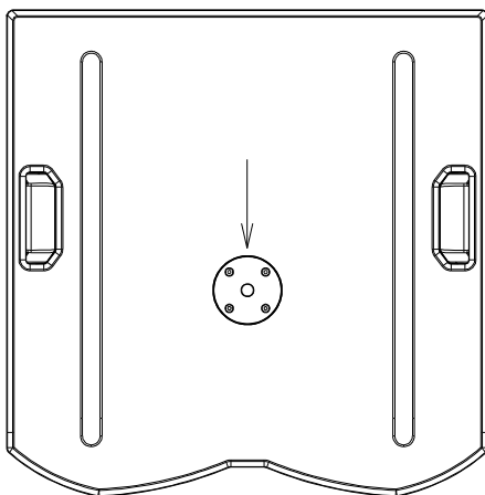
Fig. 9. S18W socket
