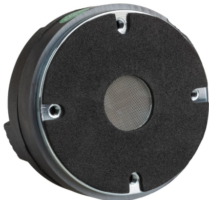
Hauptansicht – Frontansicht (1,50" Titanmembran)
