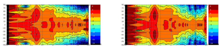
Horizontale und vertikale Isobaren in
